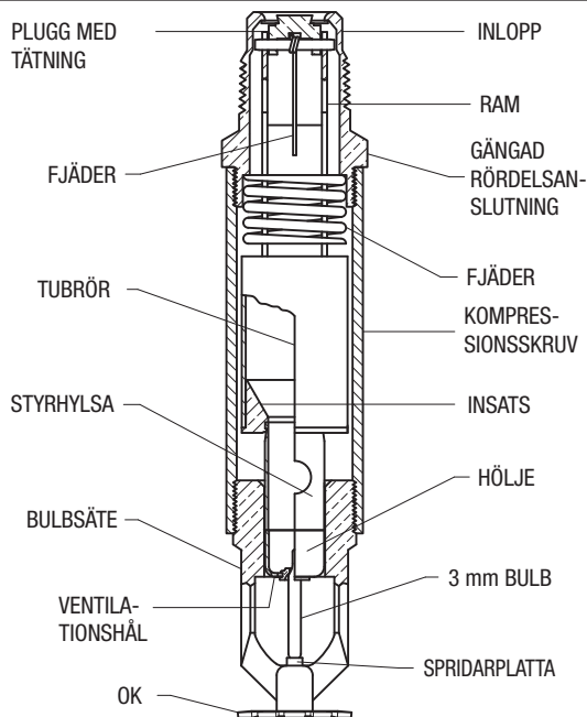
FIGUR 1 SERIE DS-1, 3/4\"/>
